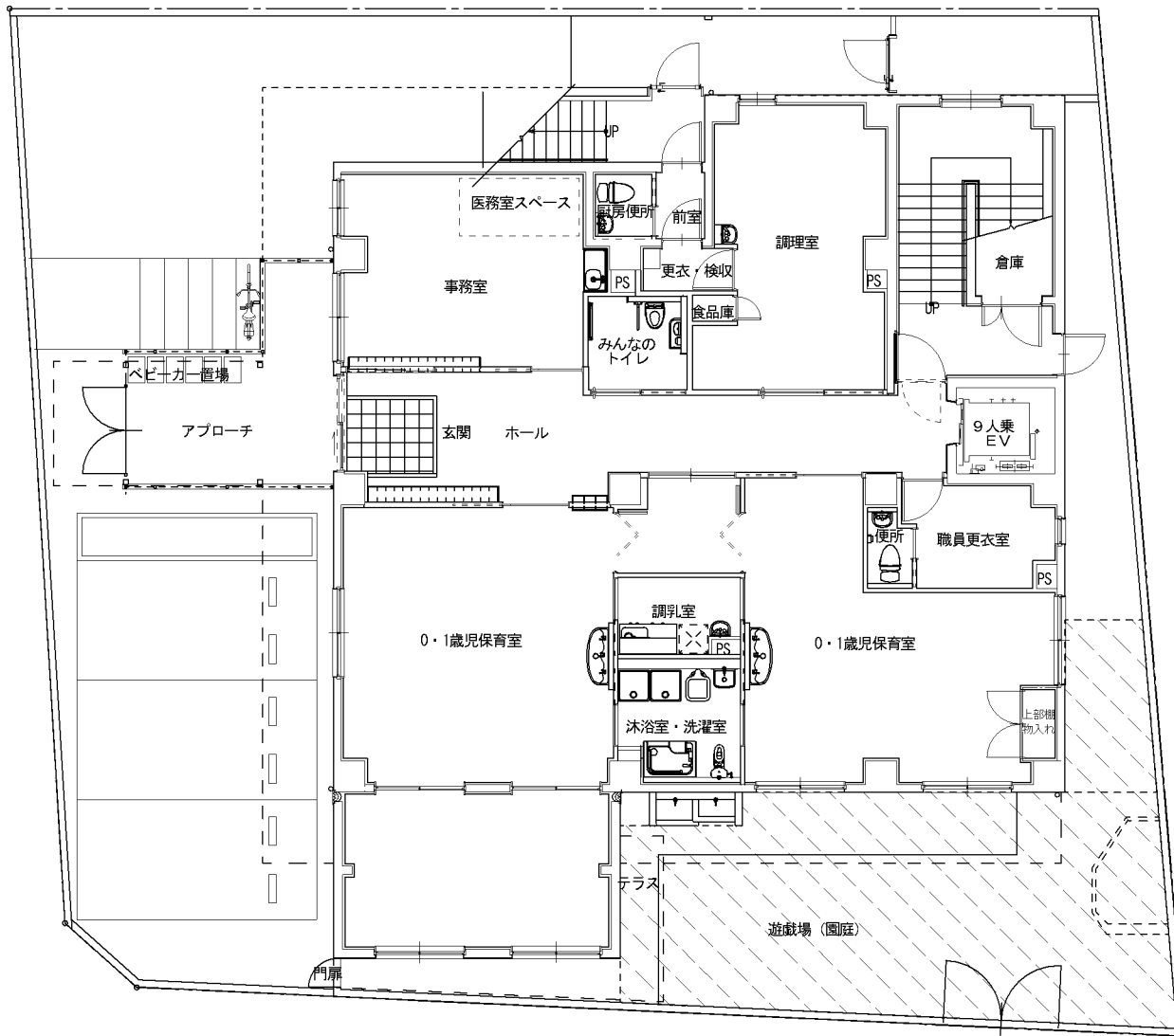
1階 平面図
