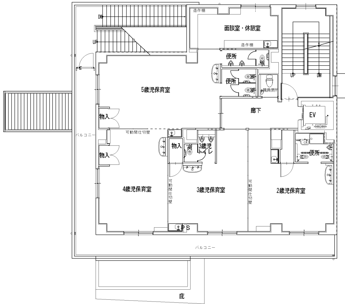
2階 平面図
